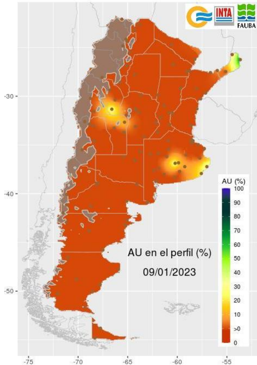
Reservas hídricas de perfil (%)
