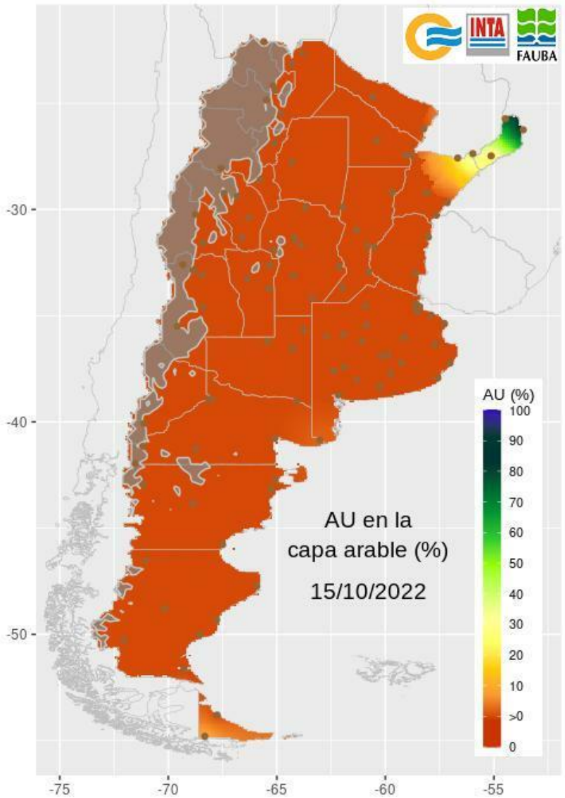
Humedad en capa arable (%)
